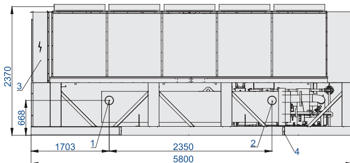
Вид спереди
