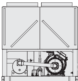
Вид слева
