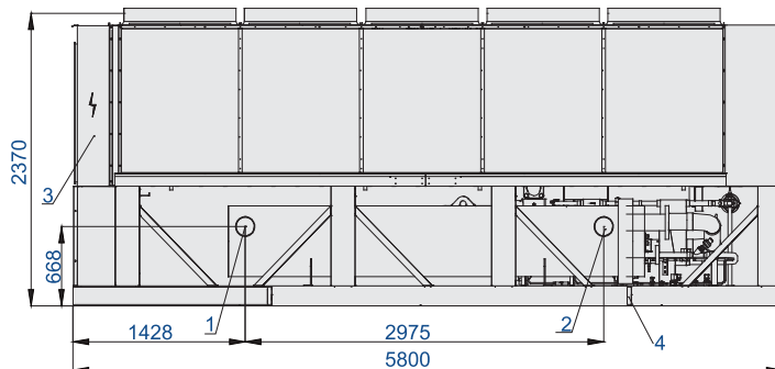
Вид спереди
